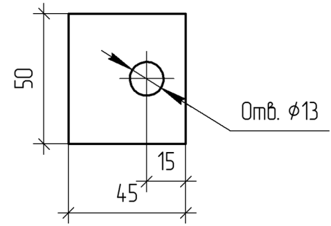
Поз 2 М 1:2
