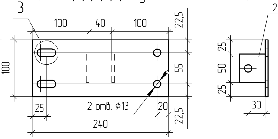
Поз 2 М 1:2
