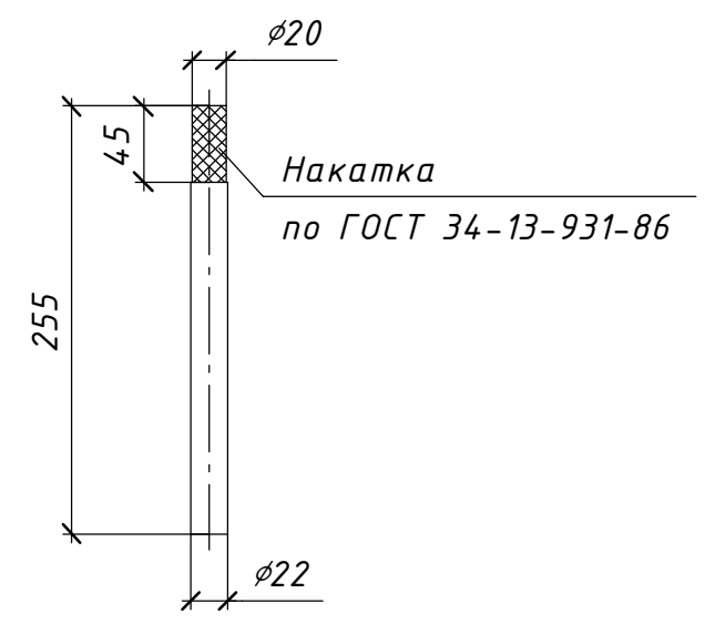
Поз. 4 (1:5)
