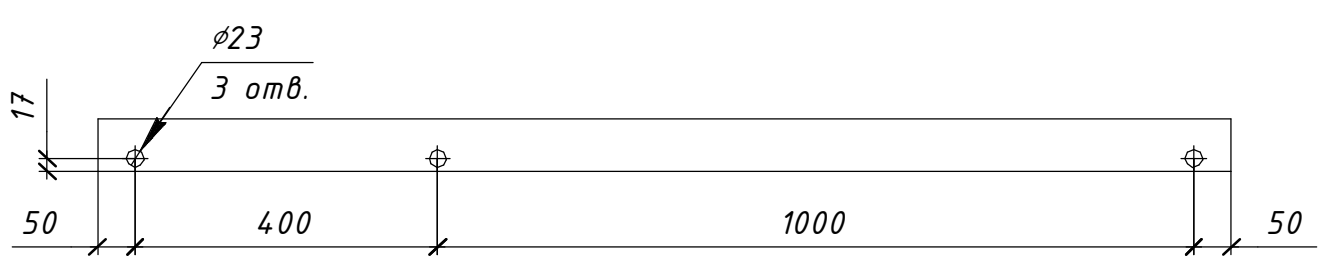
Поз. 4 (1:5)
