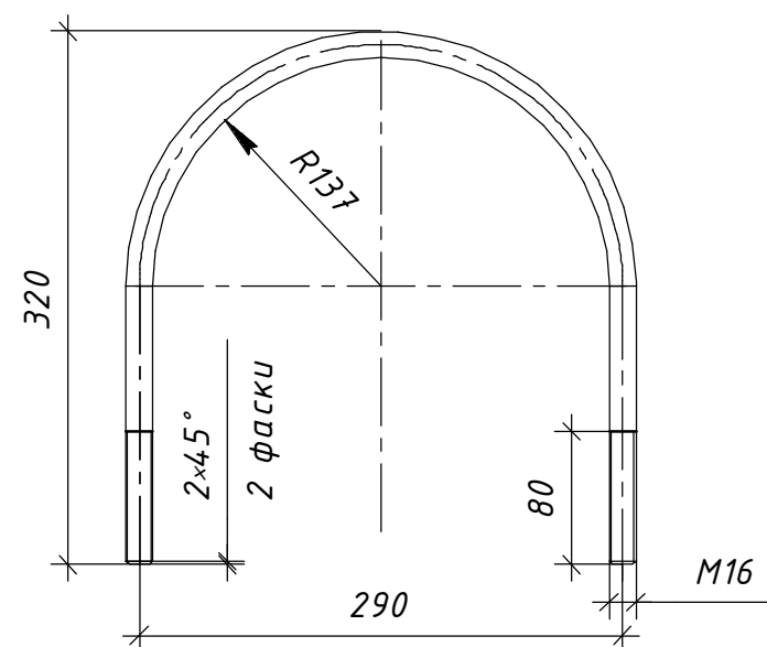
Поз. 3 (1:5)
