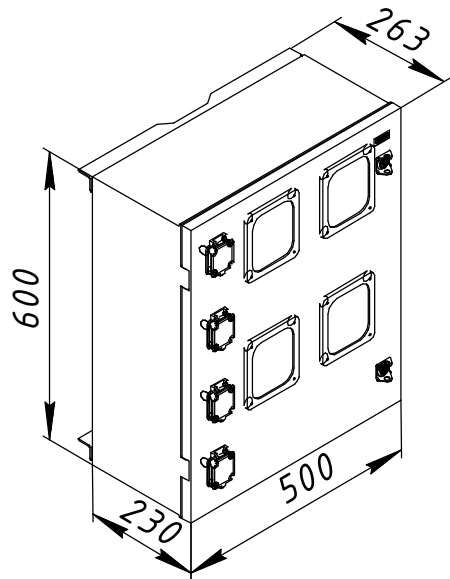
Шафа ARED-65-M4
