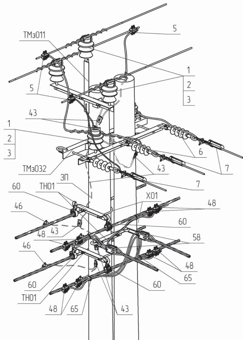
Тип стояка в залежності від тяжіння T_{max} та кількості ліній ПЛІ 0,38 кВ
