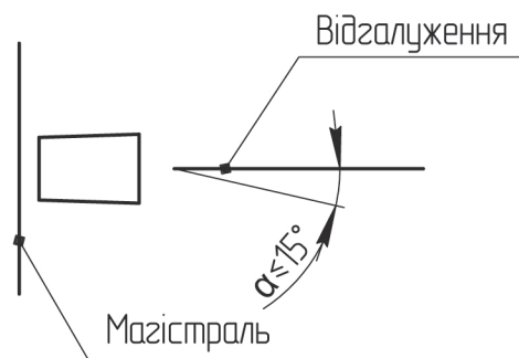
Схема встановлення опори
