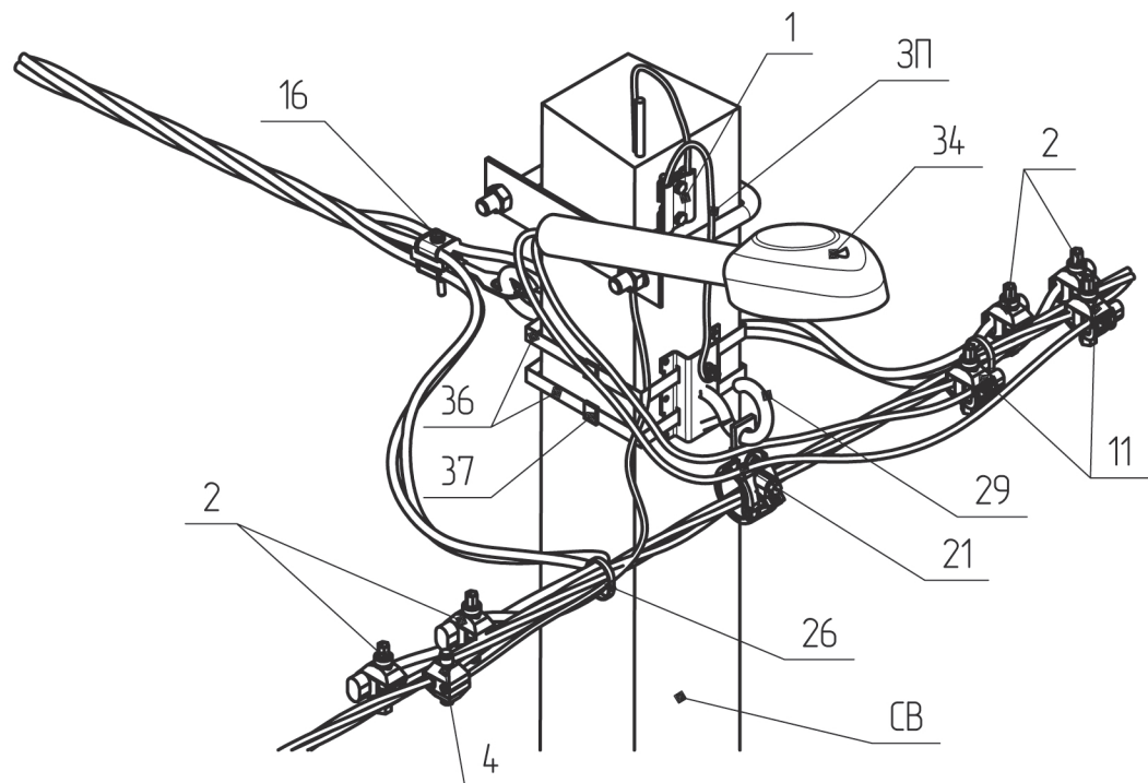
Схема встановлення опори
