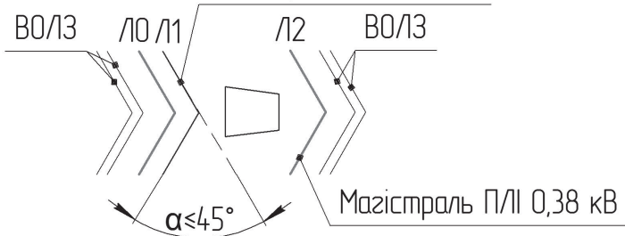
Схема встановлення опори Магістраль ПЛ 0,38 кВ
