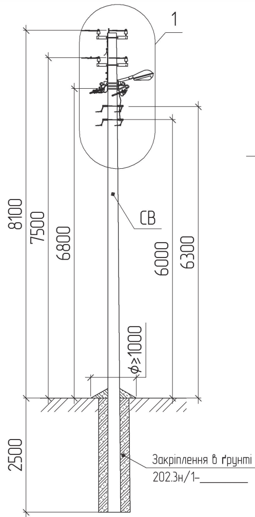
Схема встановлення опори Магістраль ПЛ 0,38 кВ
