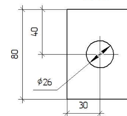
Поз 6 М 1:2
