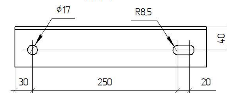
Поз 3 М 1:4
