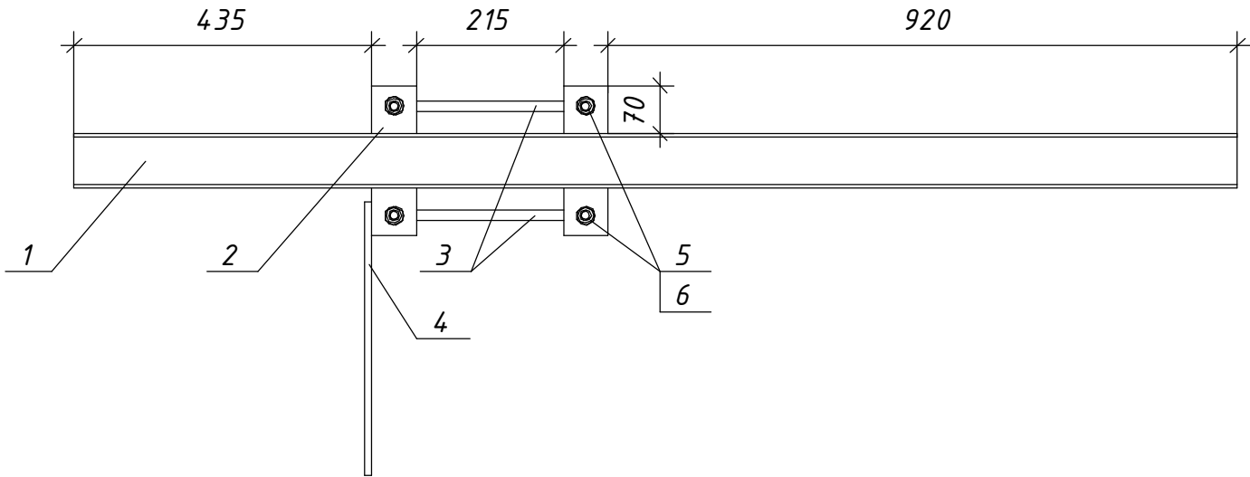
Поз. 2 (1:5)
