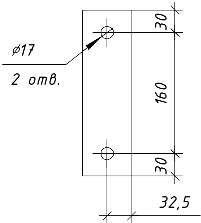
Поз. 2 (1:5)
