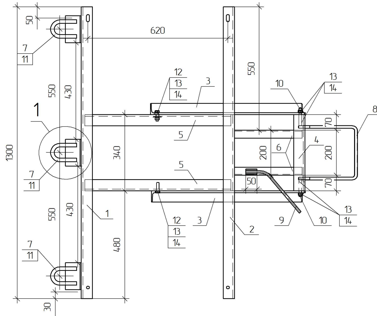
Вид А
