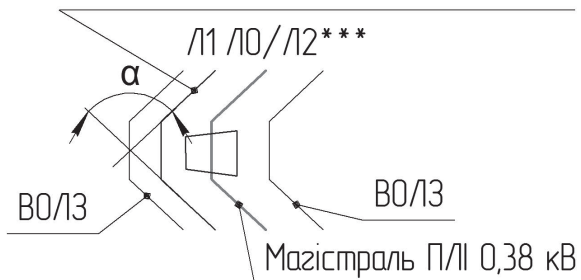
Схема встановлення опори Магістраль П/Л 0,38 кВ ( T_{max}=0,5кН )
