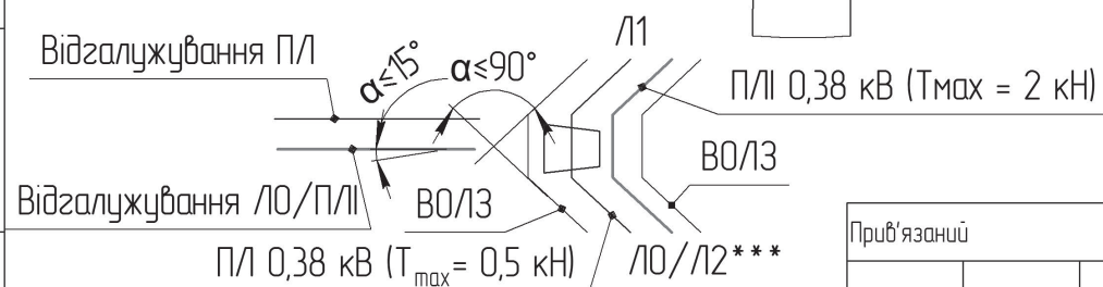
Схема встановлення опори
