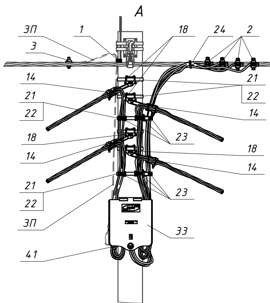
Схема підключення до Multibox DB2-4
