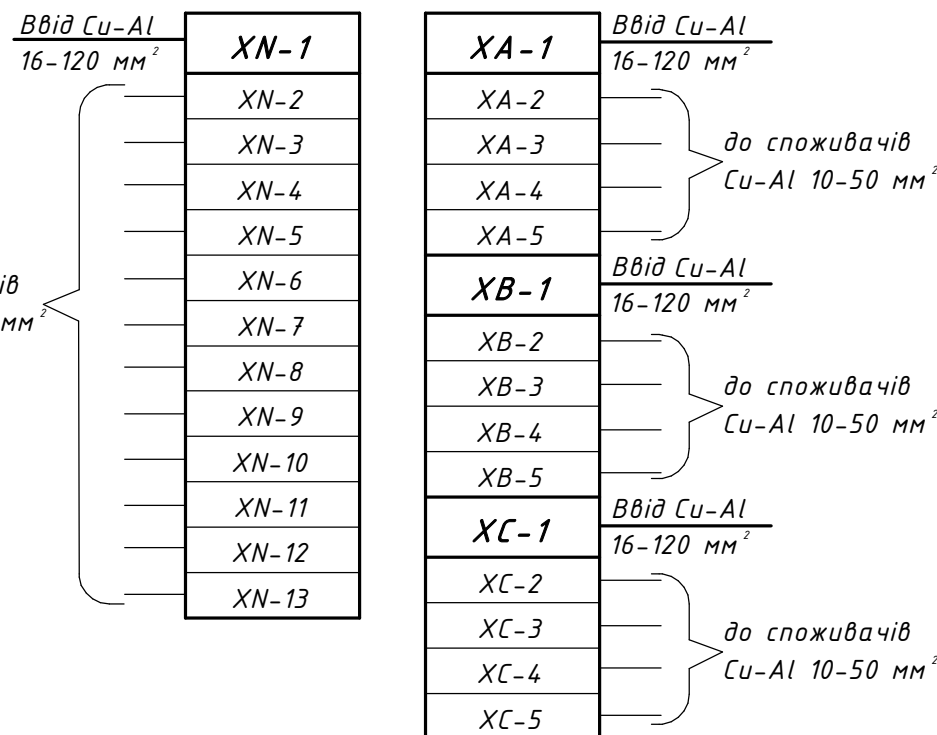
Схема підключення до Multibox DB2-4
