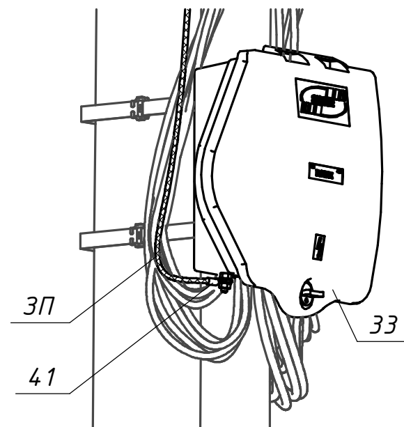
Підключення PEN-провідника
