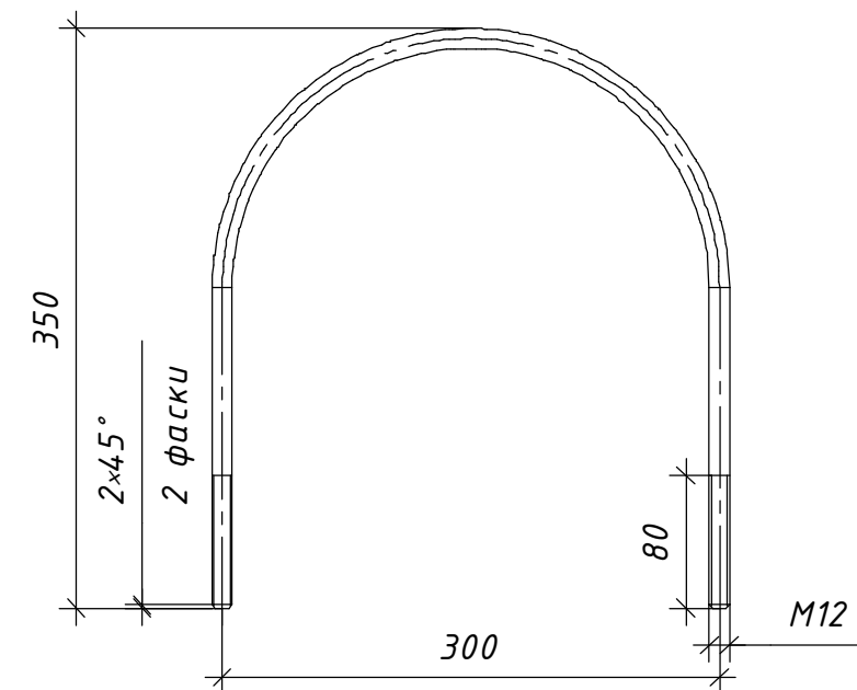
Поз. 5 (1:5)
