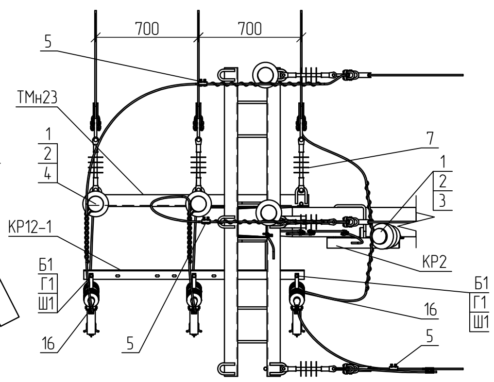
Вид А
