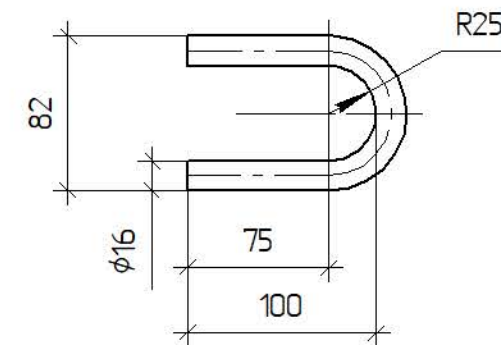
Поз 3 М 1:4
