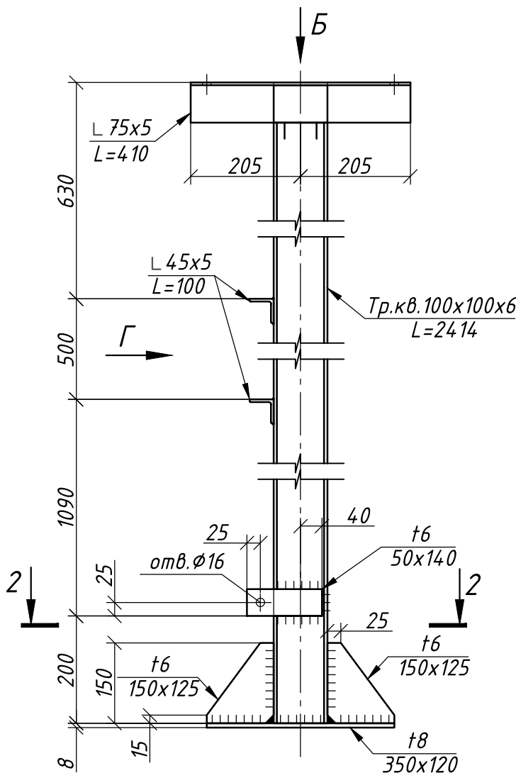
Стійка Ст1н
