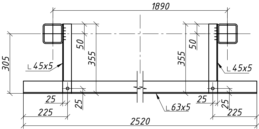
2 - 2 (М1:10)
