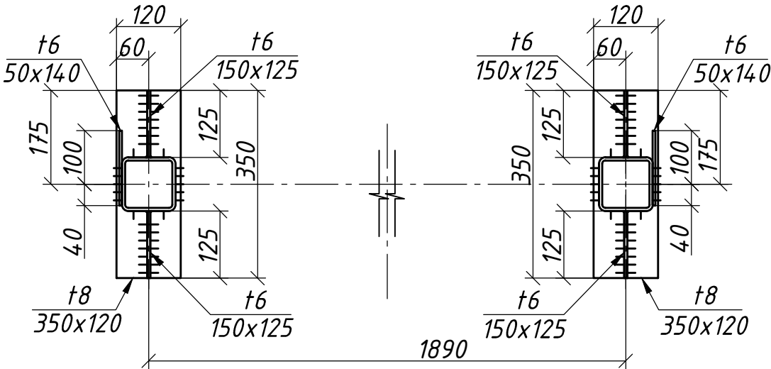
1 - 1 (М1:10)
