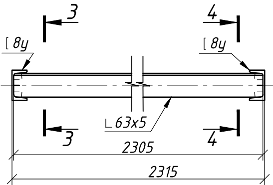
Ригель P2
