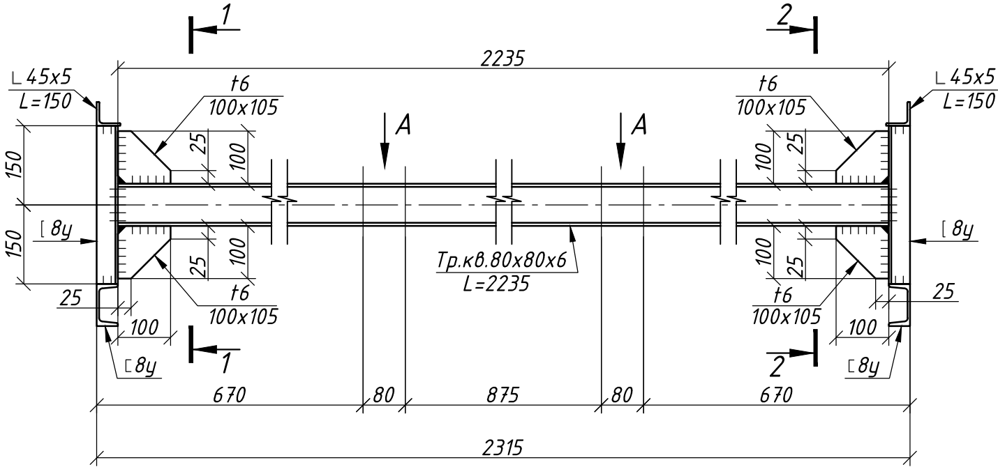
Ригель P1
