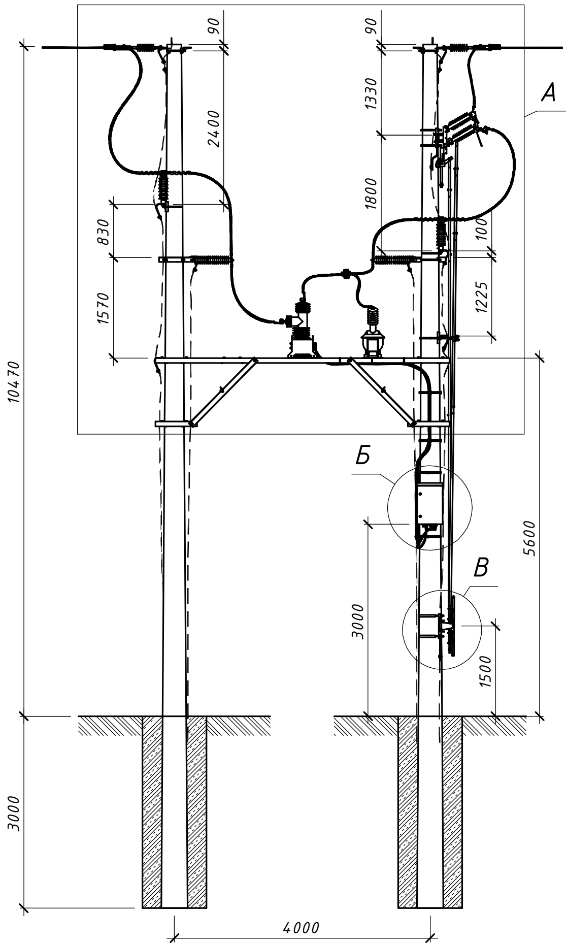
Схема встановлення опор
