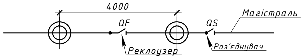
Схема встановлення опор
