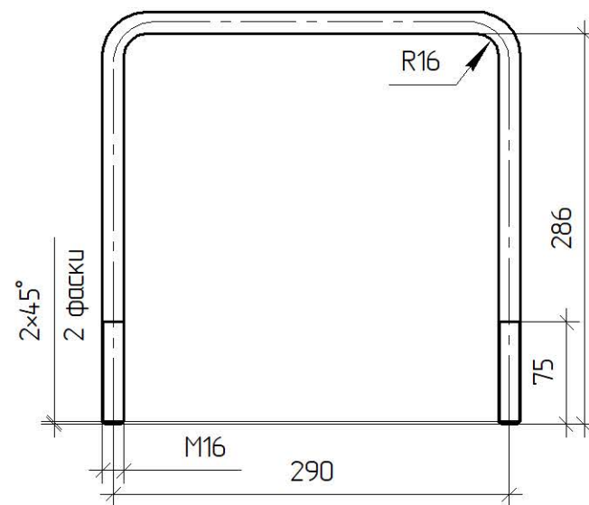
Поз 4 М 1:4
