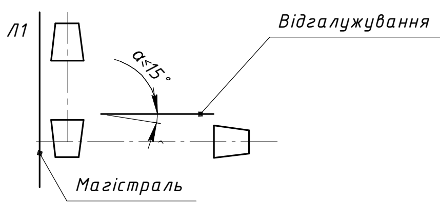
Схема встановлення опори
