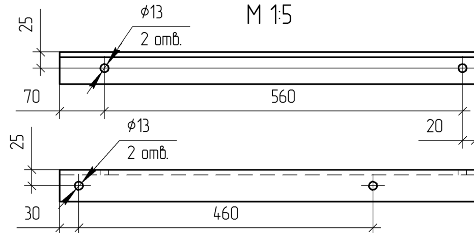
Поз 2 М 1:5
