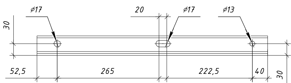
Поз. 2 (1:5)
