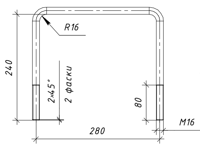
Поз. 5 (1:5)
