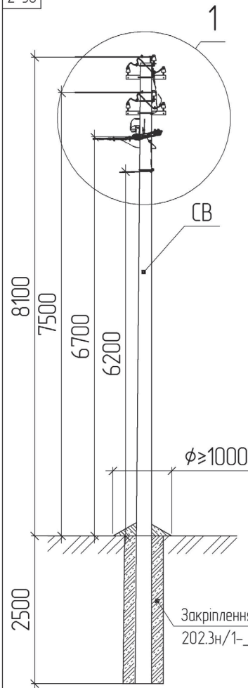
Схема встановлення опори
