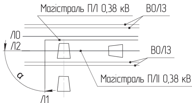
Схема встановлення опори
