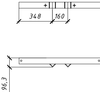
Поз. 3 та Поз. 7 (1:20)
