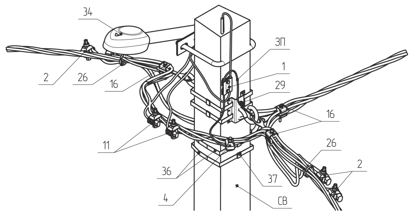
Схема встановлення опори Магістраль
