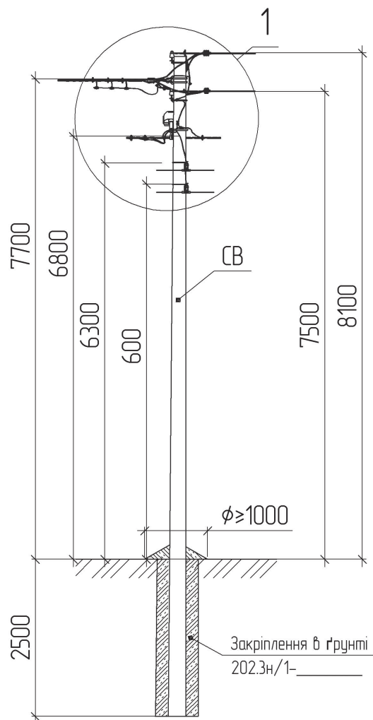
Схема встановлення опори Магістраль П/Л 0,38 кВ ( T_{\max} = 0,5 кН)
