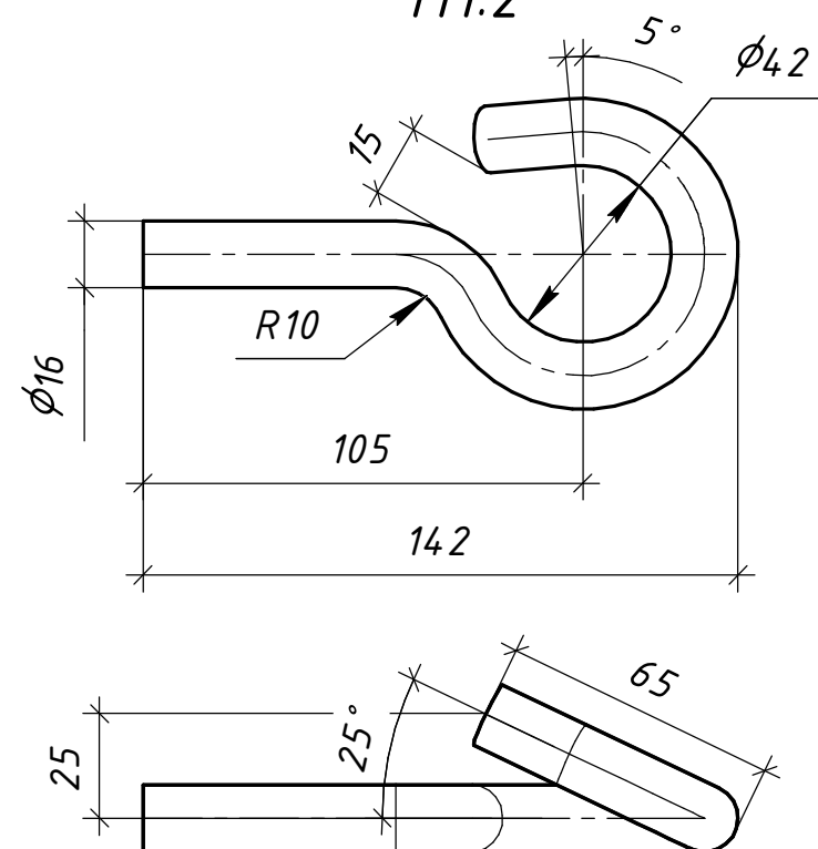
Поз 2 М1:2
