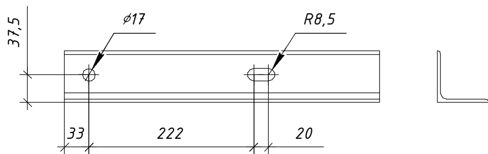
Поз. 2 (1:5)
