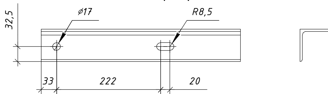
Поз. 3 (1:5)
