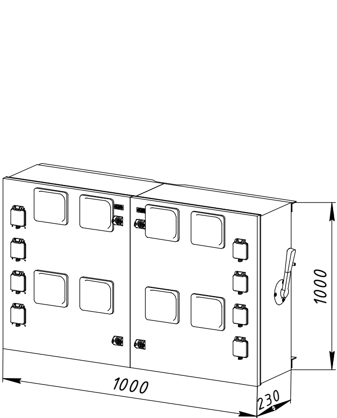
виконання Г - горизонтальне
