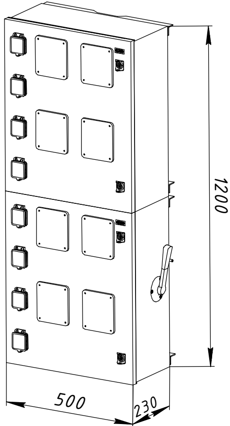
виконання В - вертикальне
