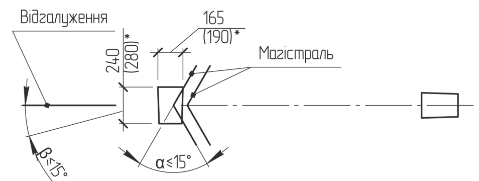
Схема встановлення опори
