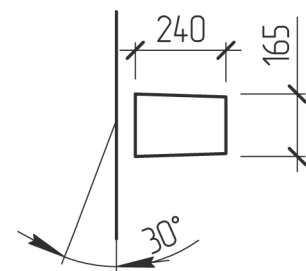
Схема встановлення опори
