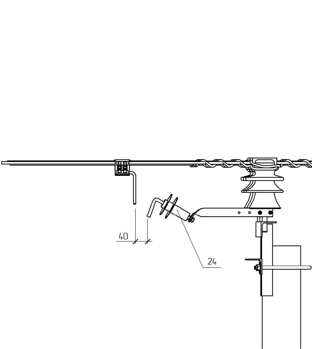
Комплект захисту П/З від атмосферних перенапруг ASICS 150и поз. 24
