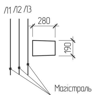
Схема встановлення опори
