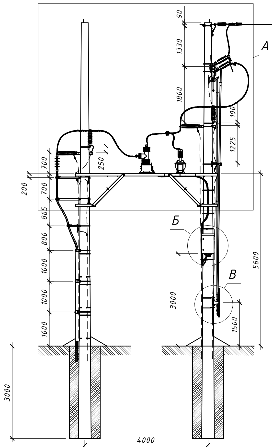
Схема восстановления опор
